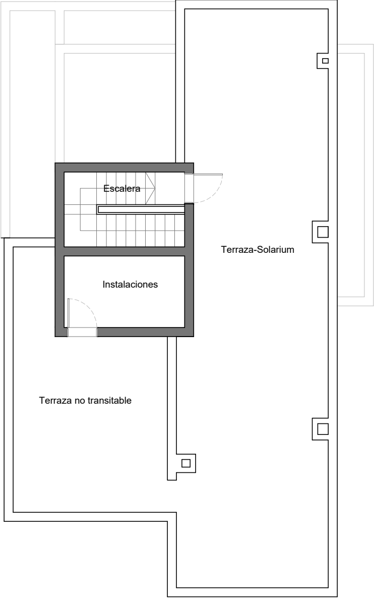
Planta cubiertas
